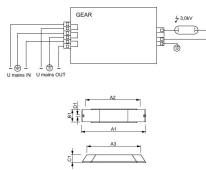
Caractéristiques Philips HID-PV m 20 /I CDM HPF 50/60Hz
